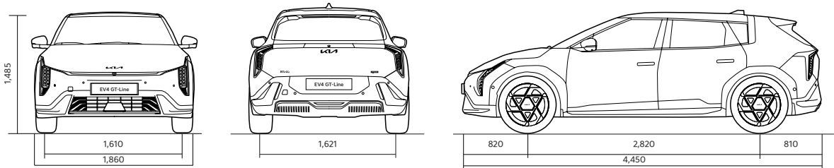
Afmetingen Hatchback GT-Line
